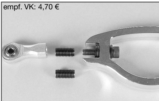
Best.-Nr./ Item N°: 6498/3 Gewindeinsatz M8/M6, 2 St. Thread insert M8/M6, 2 pcs.
