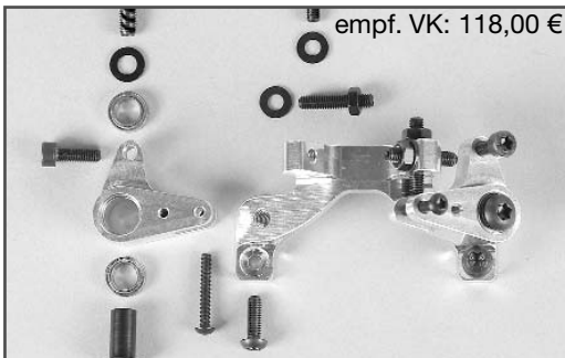
Best.-Nr./ Item N°. 10353 Dämpferumlenkung vorne kugelgel. für F1 Competition, Set Front damper reversing ball-bearing for F1 Competition, set
