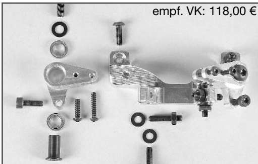
Best.-Nr./ Item N°. 10363 Dämpferumlenkung hinten kugelgel. für F1 Competition, Set Rear damper reversing ball-bearing for F1 Competition, set
